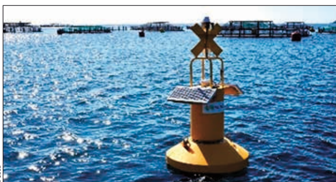
L'une des deux bouées technologiques prochainement mises en place à Cannes : ici celle de Suez, capable de mesurer les bruits anthropiques.
